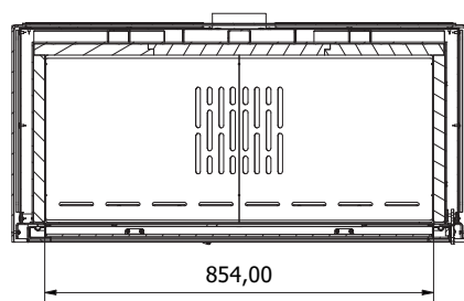
G-G ( 1 : 10 )
